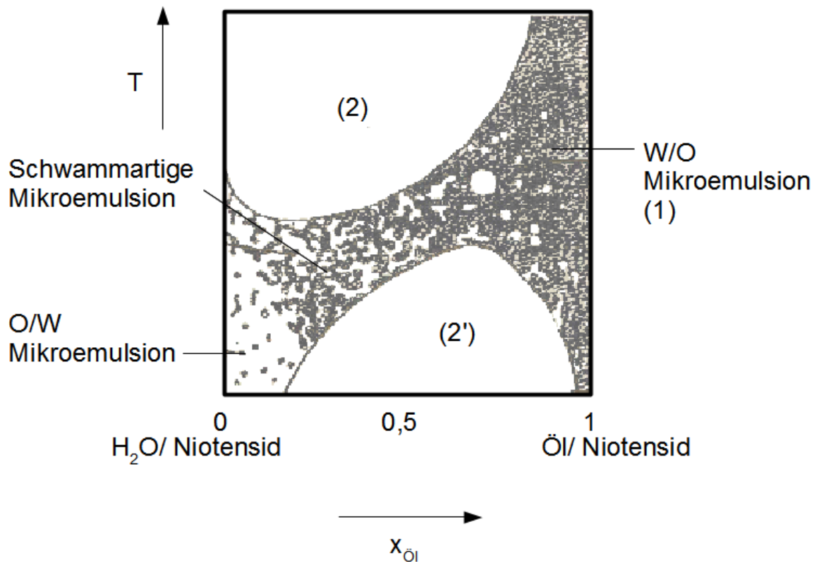
Abbildung 2.2.: Schnitt durch ein Zustandsdiagramm Wasser-Öl-Niotensid; (1) einphasiges Gebiet; zweiphasige Gebiet, das Tensid ist hier in der wässrigen (2) bzw. in der öligen (2') Phase gelöst; x Molenbruch, T Temperatur; nach [Dörfler, 2002]
