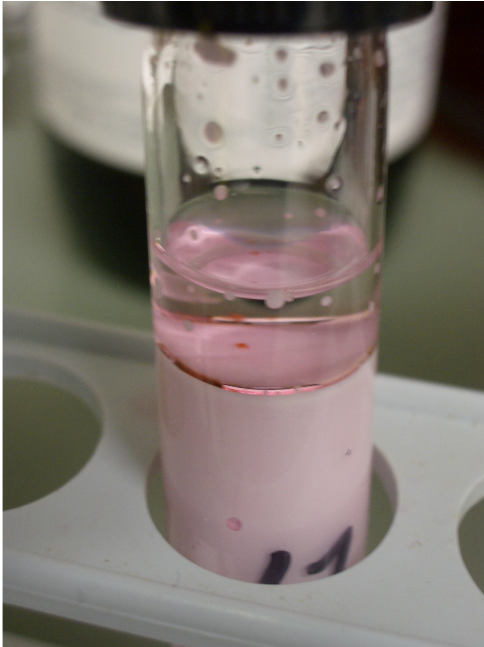
Abbildung 2.4.: Hexanol
