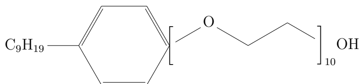
Abbildung 2.4.: Strukturformel Igepal
