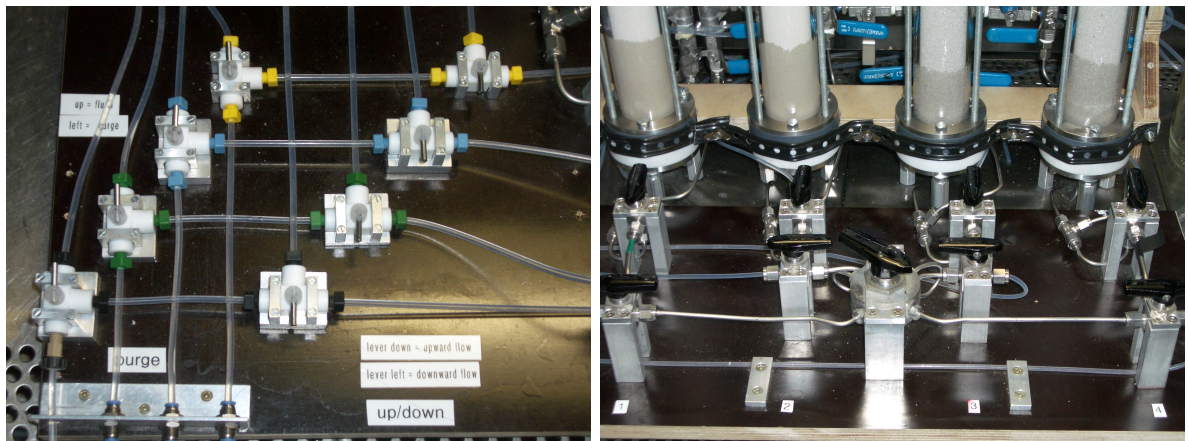
(a) Dreiwegeventile zur Steuerung des Zulaufs
