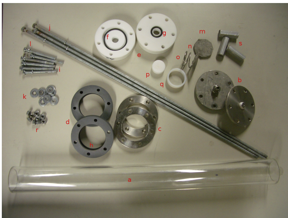
Abbildung 3.5: Säulenzubehör
