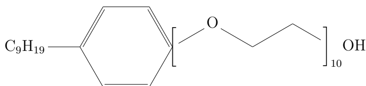
Abbildung 3.4: Strukturformel Igepal
