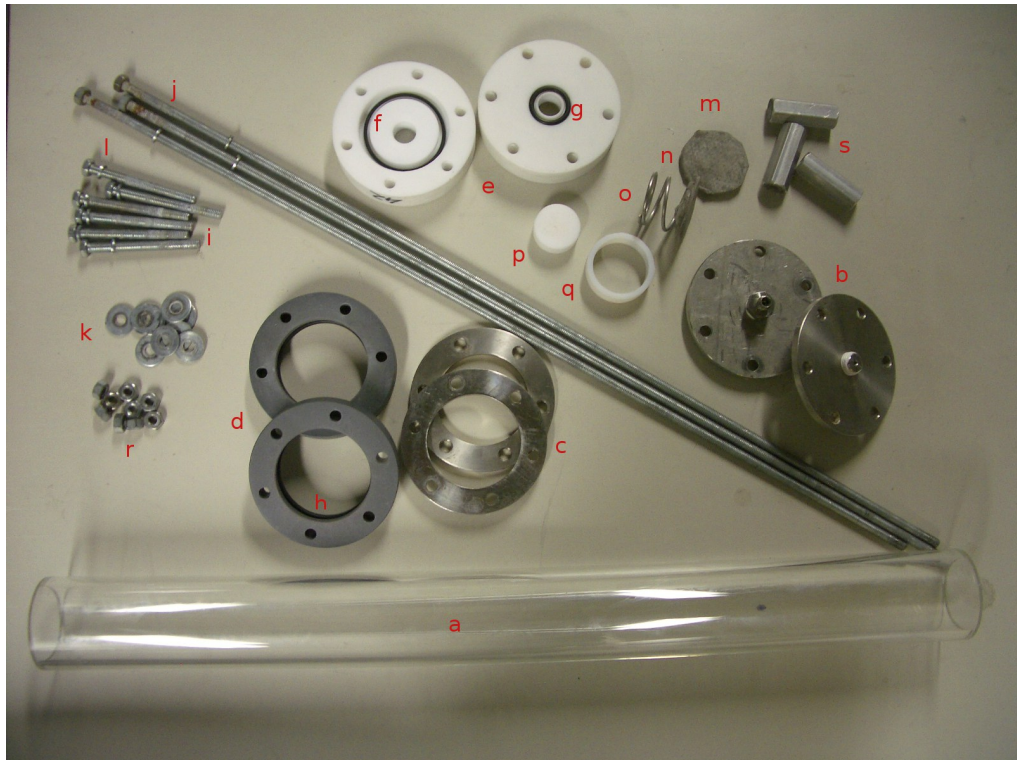
Abbildung 3.5: Säulenzubehör
