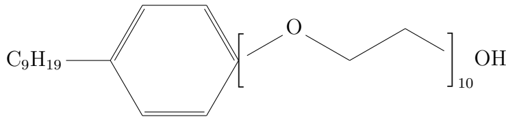
Abbildung 3.4: Strukturformel Igepal
