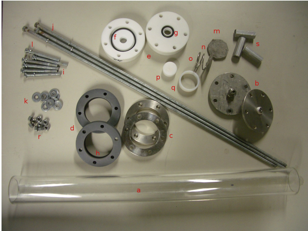
Abbildung 3.5: Säulenzubehör
