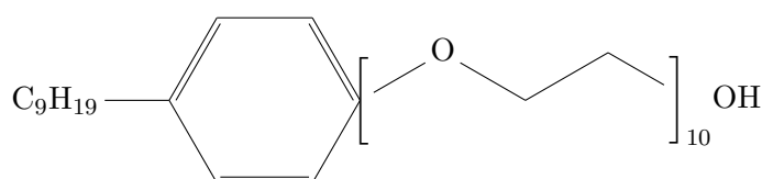
Abbildung 3.4: Strukturformel Igepal
