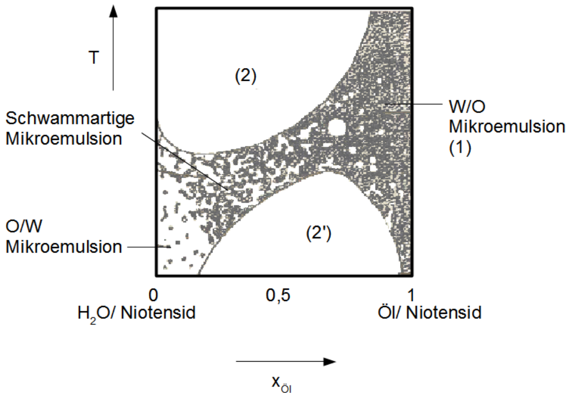
Abbildung 2.2: Schnitt durch ein Zustandsdiagramm Wasser-Öl-Tensid; (1) einphasiges Gebiet; zweiphasige Gebiet, das Tensid ist hier in der wässrigen (2) bzw. in der öligen (2') Phase gelöst; x Molenbruch, T Temperatur; nach Dörfler (2002)
