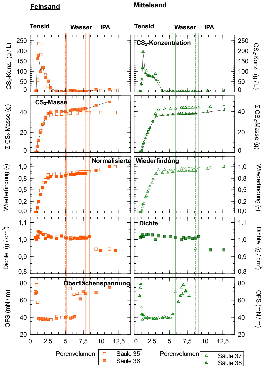
Abbildung 5.6: Säulenversuche bei 1% Tensid und einer Fließrate von 1 ml/min
