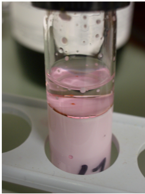
(a) Hexanol
