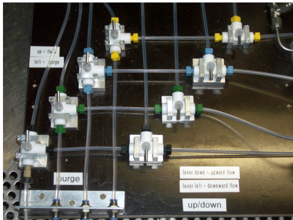
(a) Dreiwegventile zur Steuerung des Zulaufs
