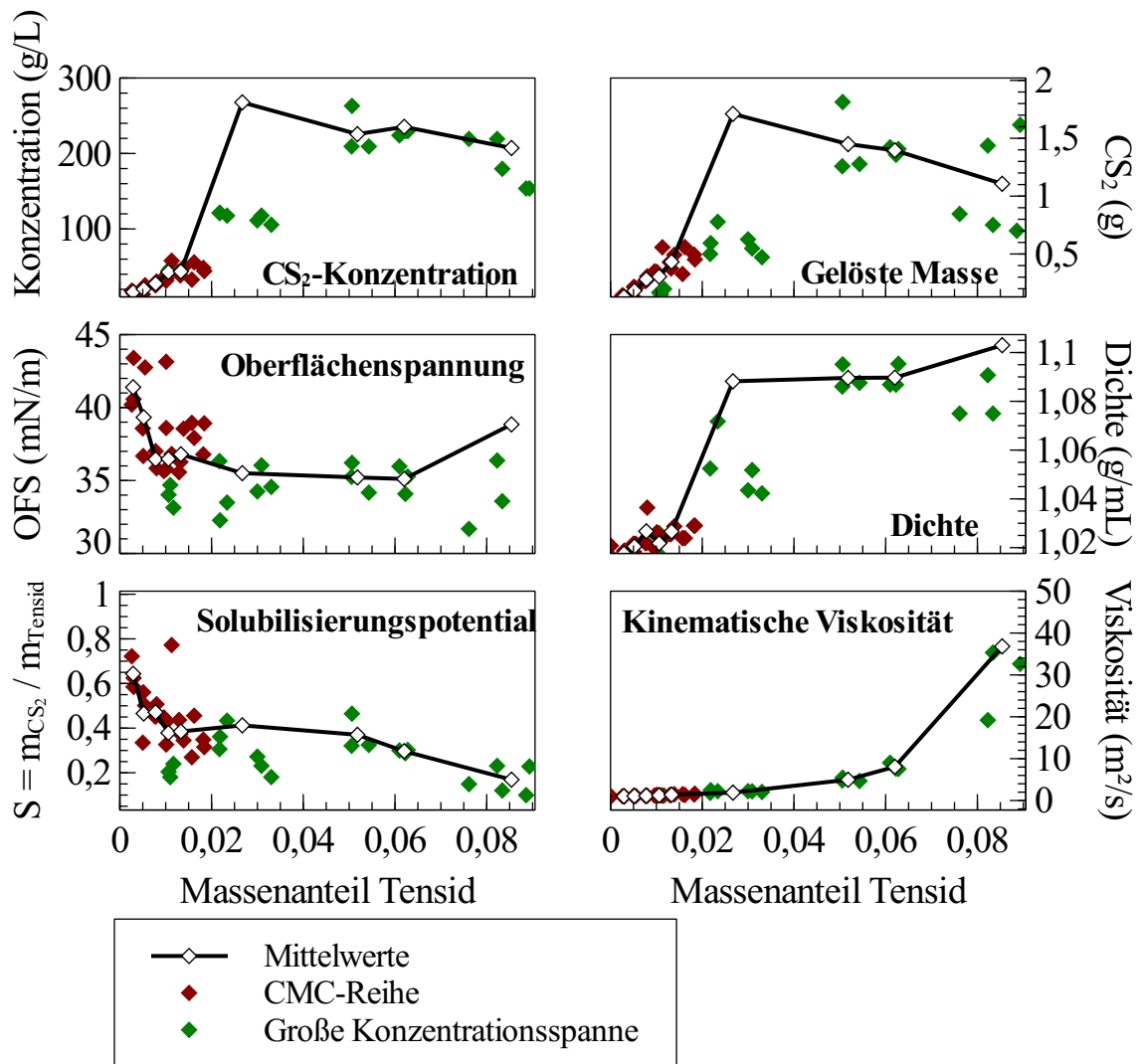
Abbildung 4.3: Messwerte der Batchversuche
