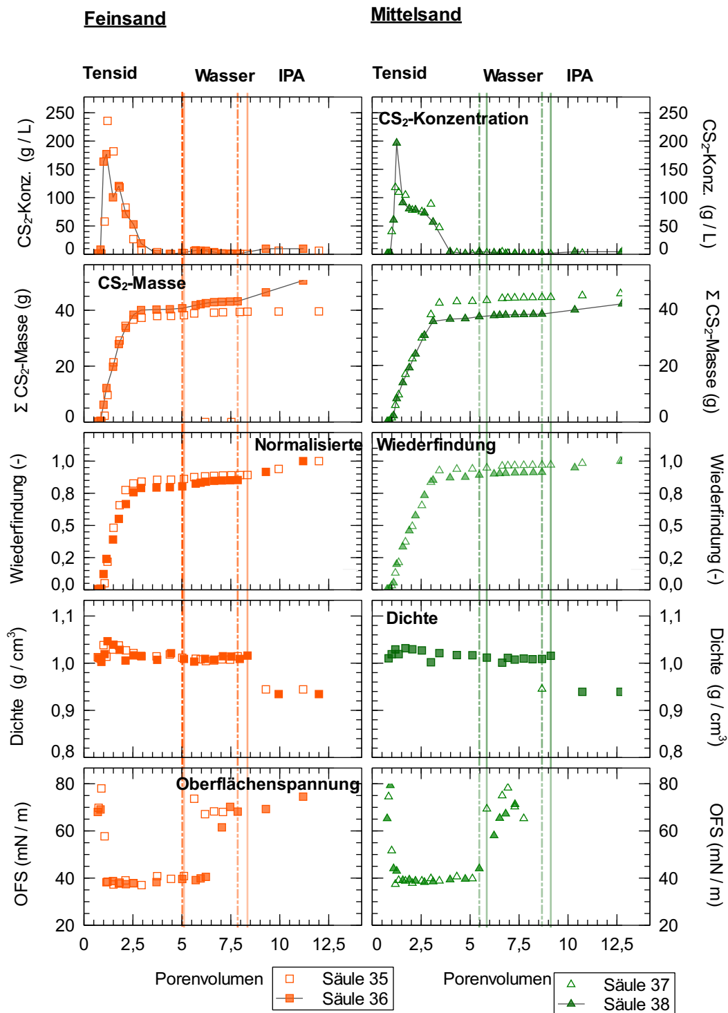
Abbildung 5.7: Säulenversuche bei 1% Tensid und einer Fließrate von 1 ml/min
