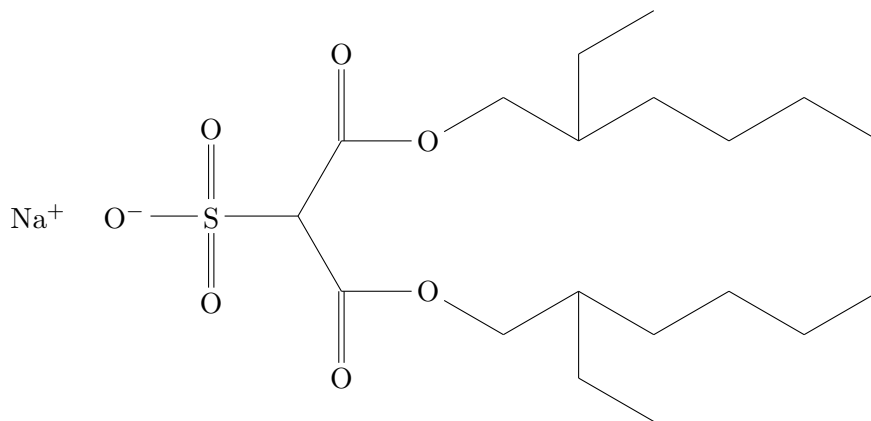
Abbildung 3.2: Strukturformel Lutensit A-BO
