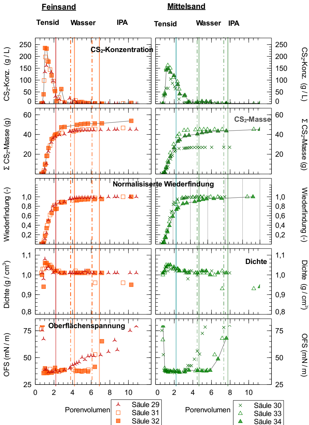
Abbildung 5.6: Säulenversuche bei 2% Tensid und einer Fließrate von 1 ml/min
