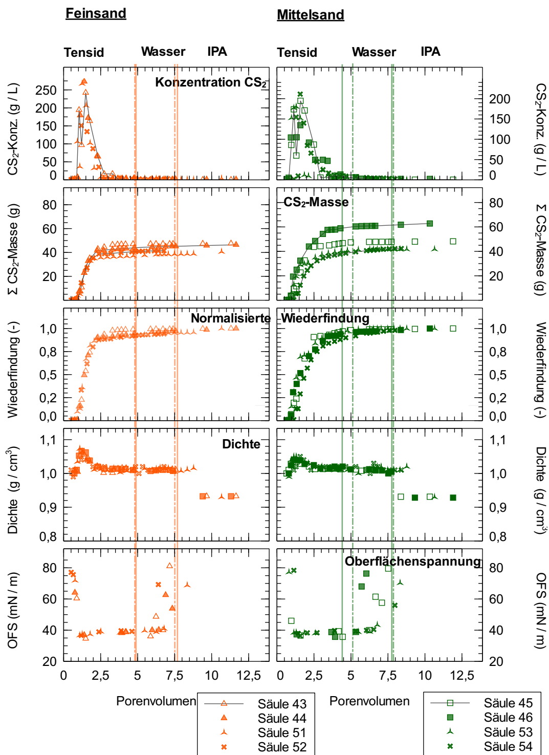
Abbildung 5.8: Säulenversuche bei 1% Tensid und einer Fließrate von 0,5 ml/min
