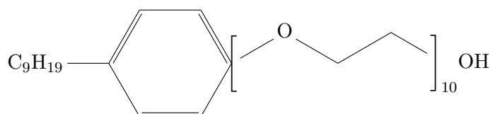
Abbildung 3.4: Strukturformel Igepal
