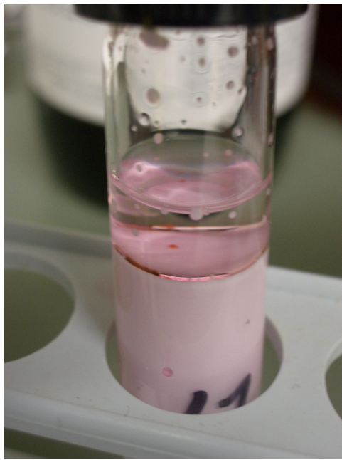
(a) Hexanol
